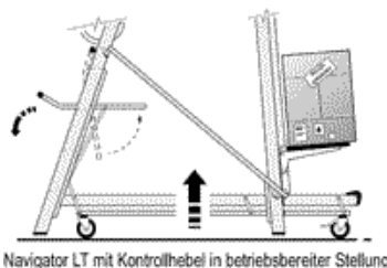
Navigator LT mit Kontrollhebel in betriebsbereiter Stellung
